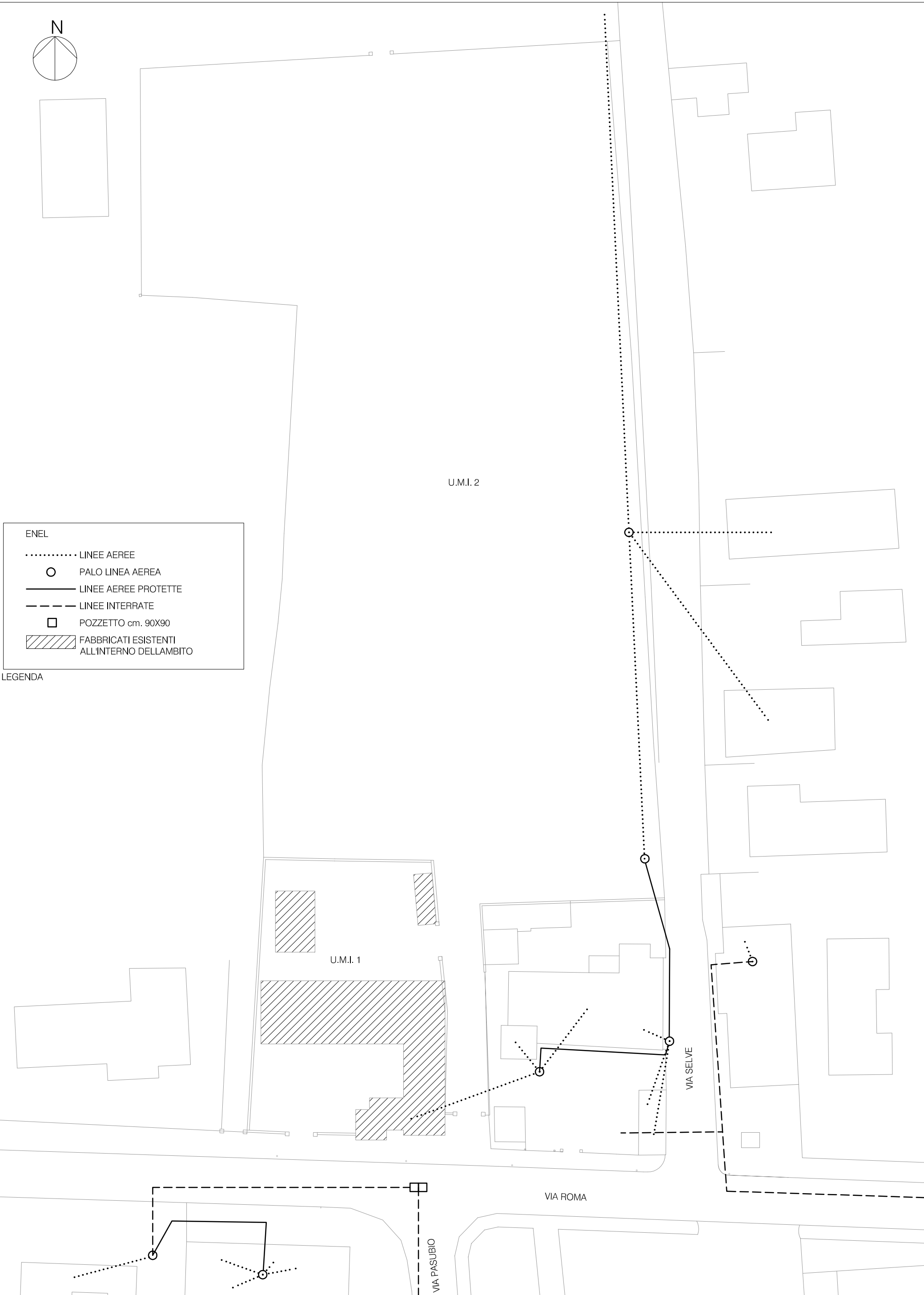
PLANIMETRIA 1:500 RETE ENEL_STATO DI FATTO
